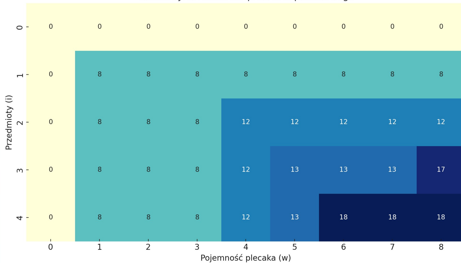
Tablica dynamiczna dla problemu plecakowego
